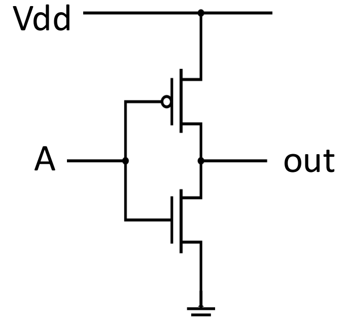
CMOS - 1983
